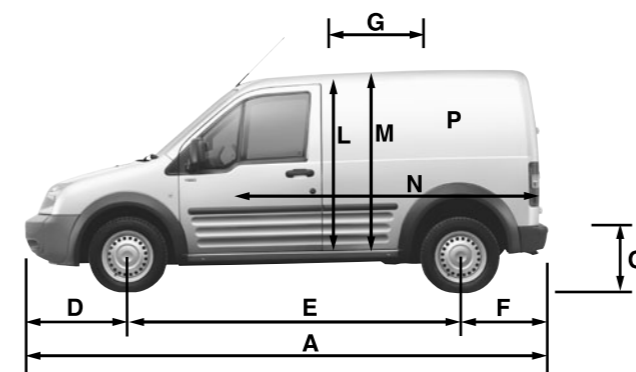
Kurzer Radstand | Empattement court | Passo corto
