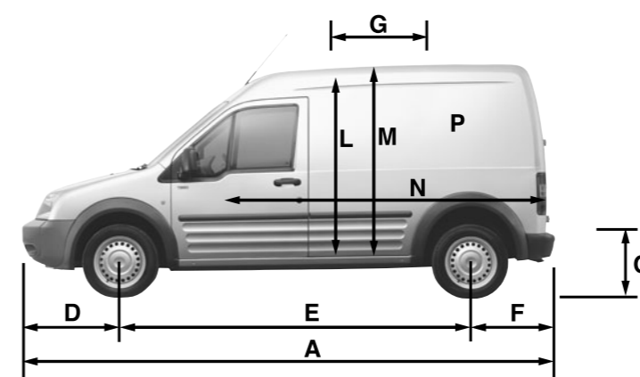
Langer Radstand | Empattement long | Passo lungo
